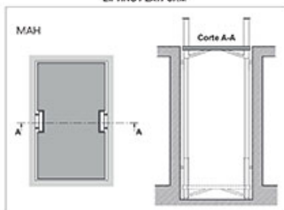
PLATAFORMA DE DUPLA COLUNA LIFTING PLATFORM
