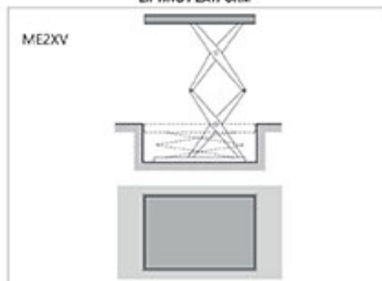
PLATAFORMA DE DUPLA TESOURA VERTICAL SCISSOR TABLE
